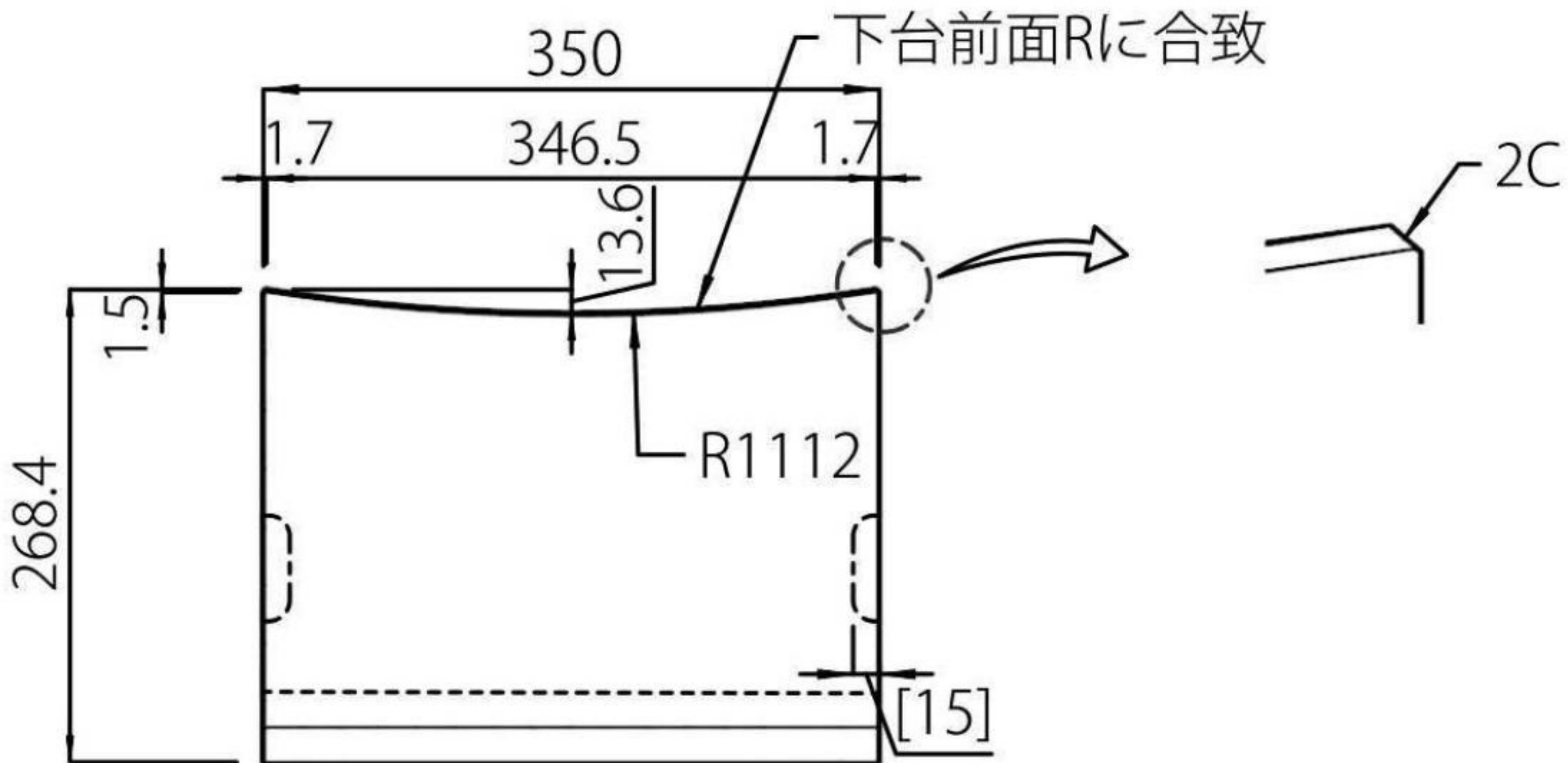
【平面図】
