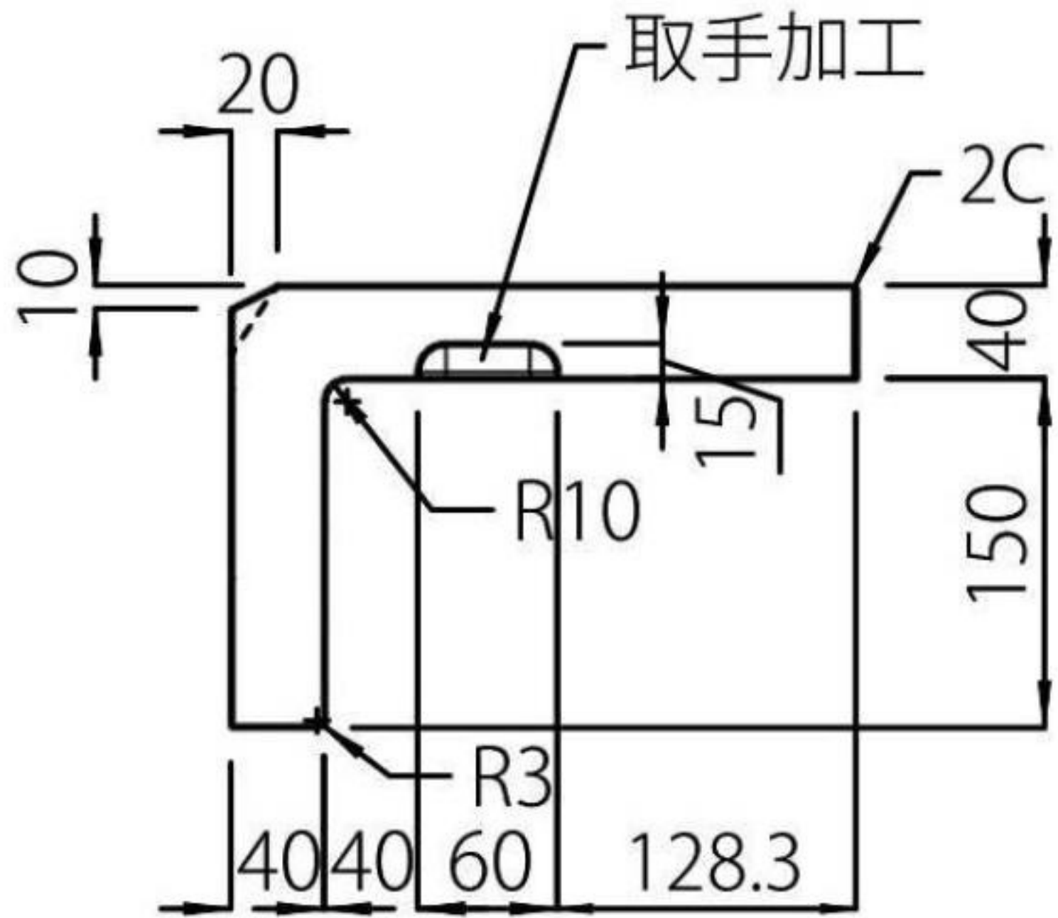
【右側面図】
