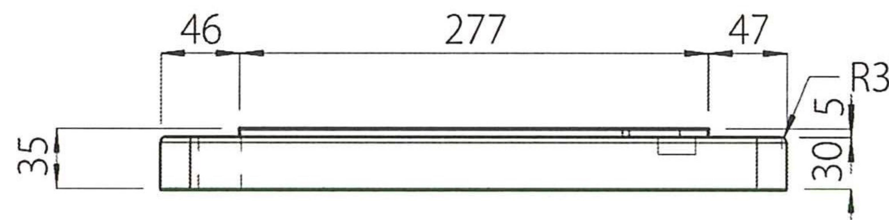
【正面図】
