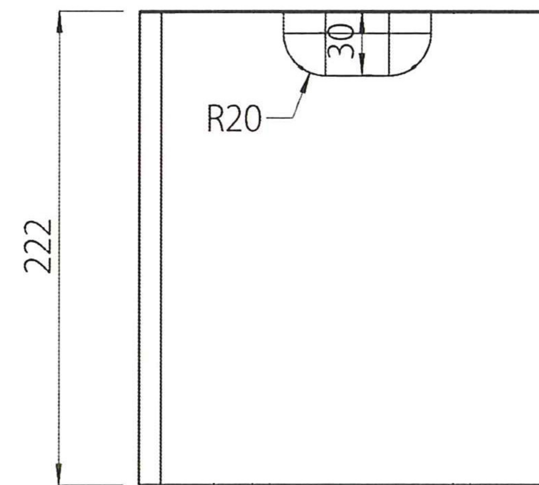
【正面図】
