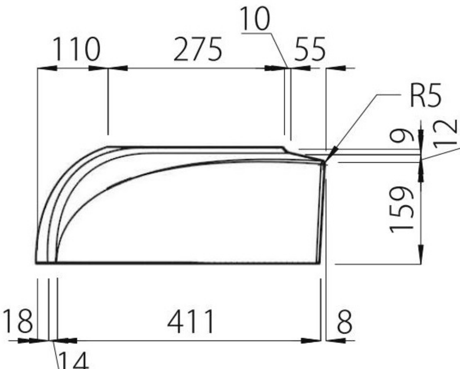
【右側面図】
