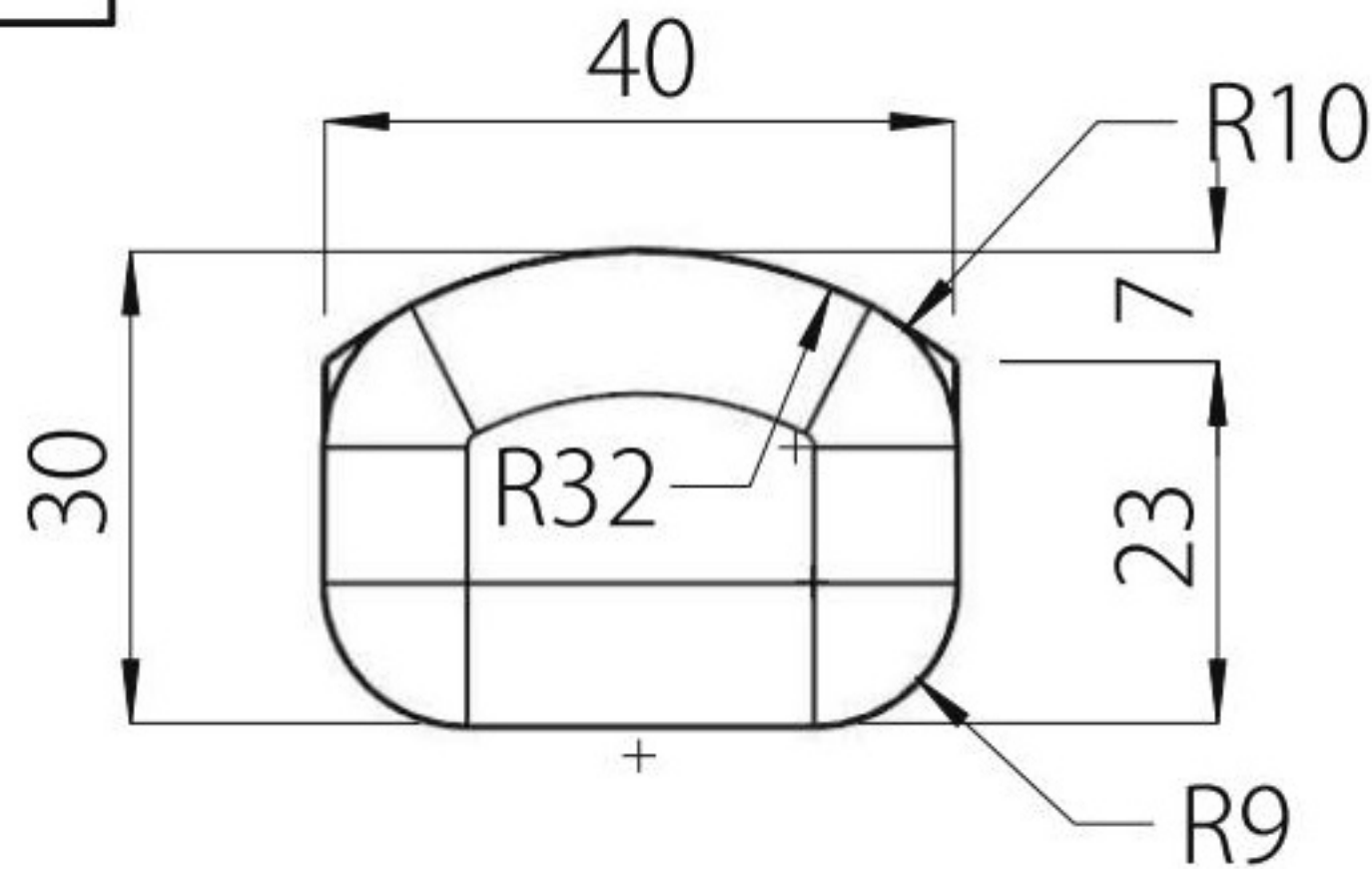
【平面図】
