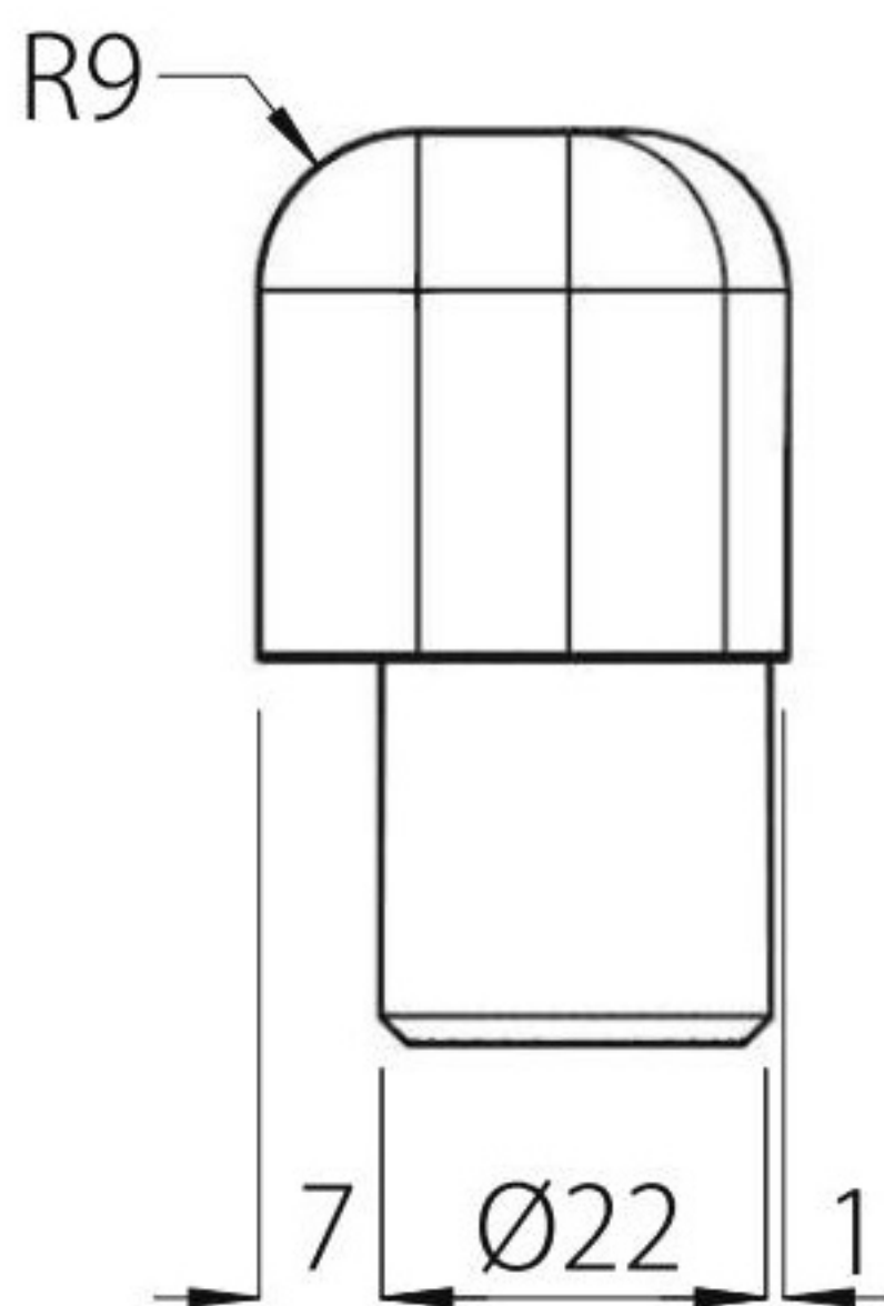
【右側面図】
