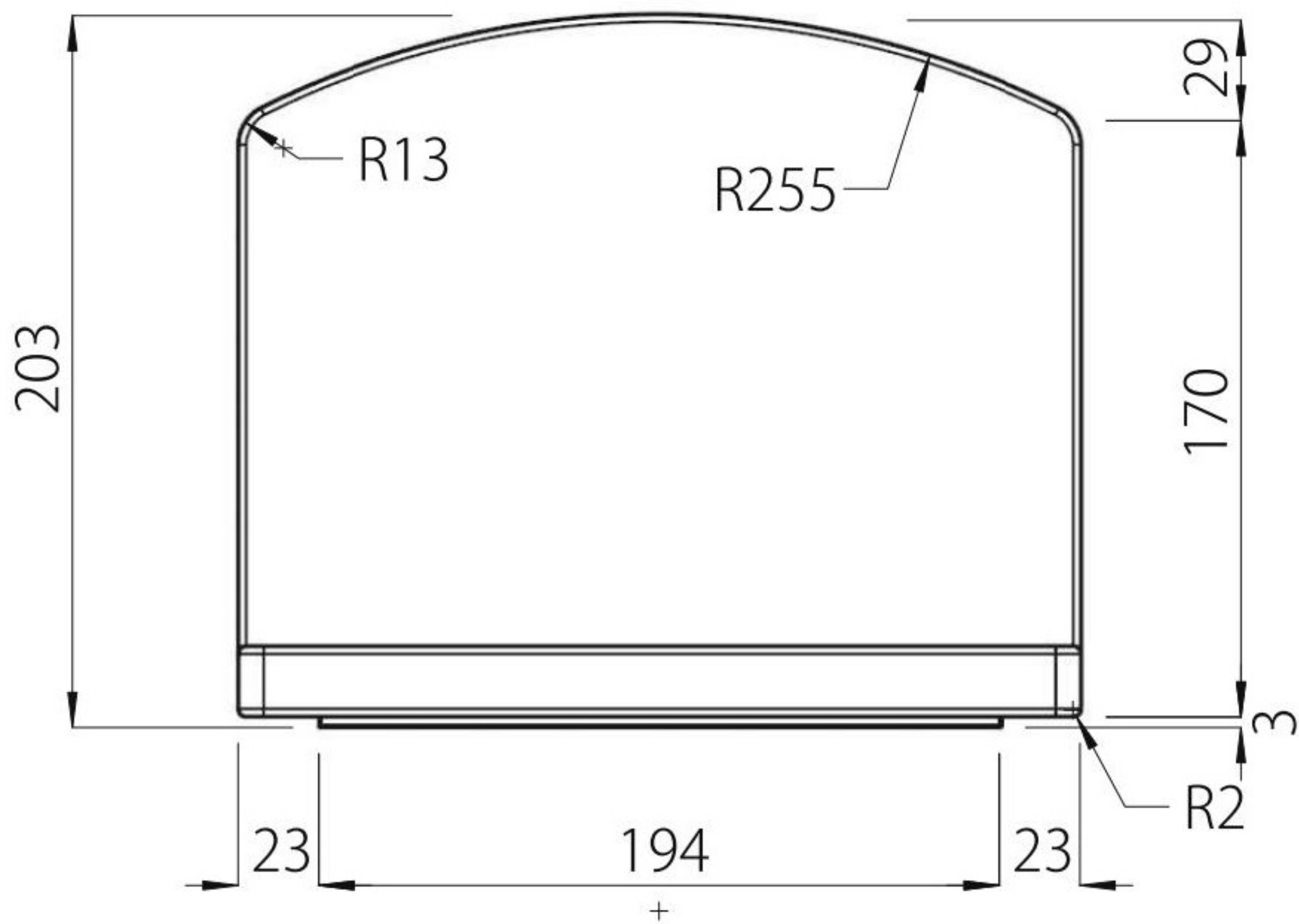
【正面図】
