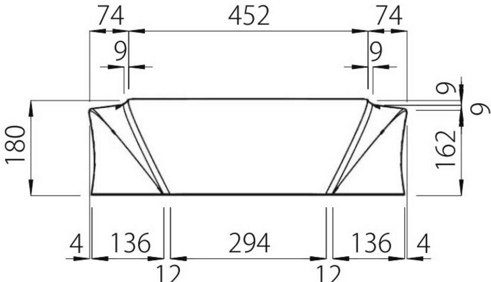
【正面図】
