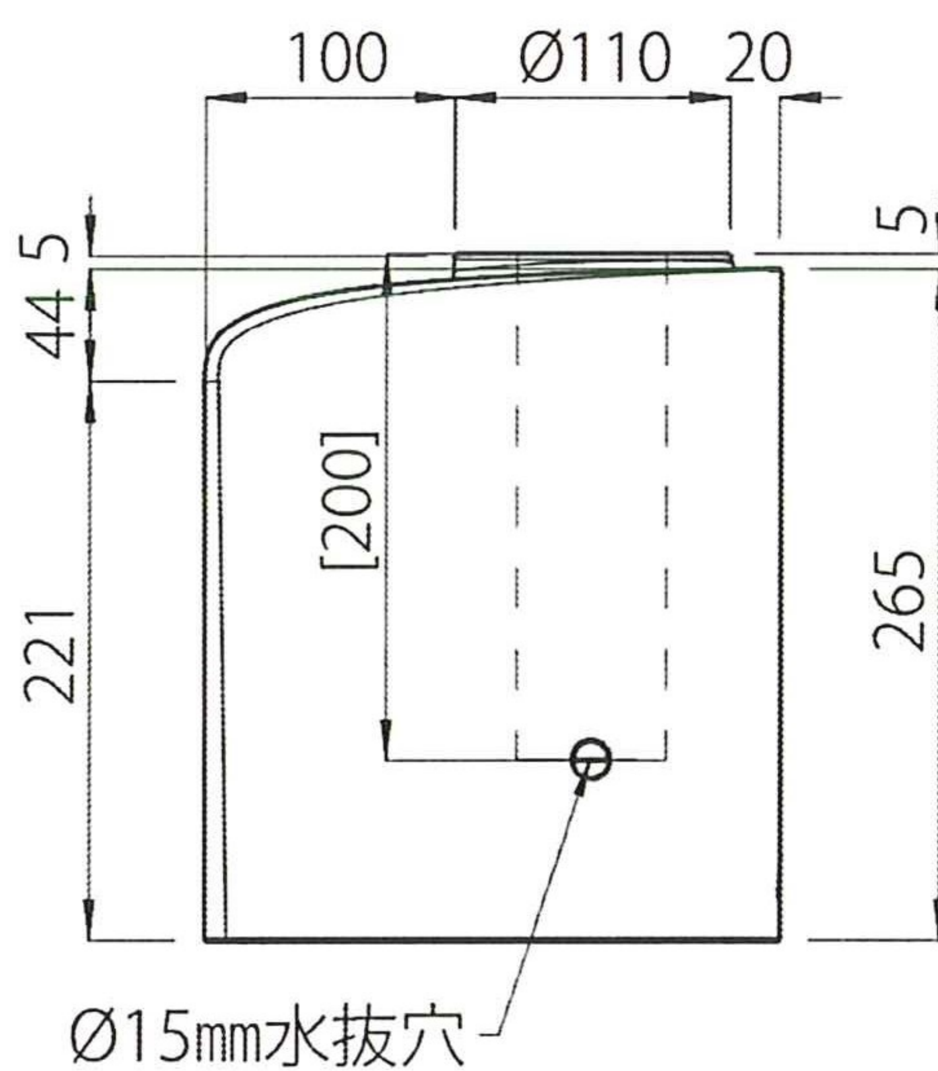
【右側面図】
