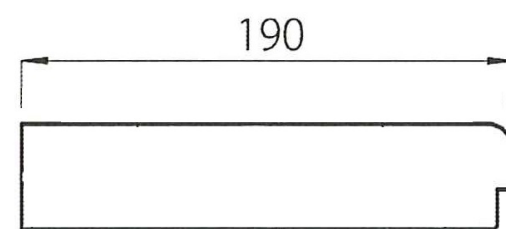
【底面図】
