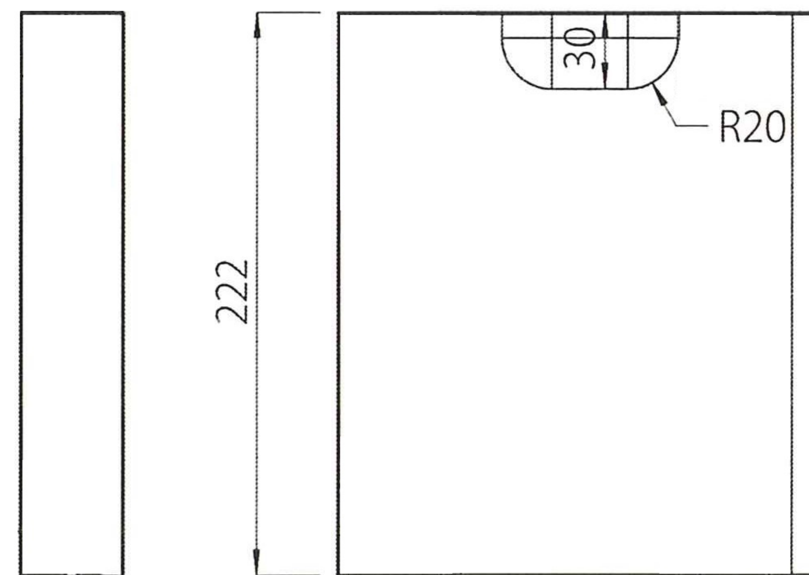
【正面図】
