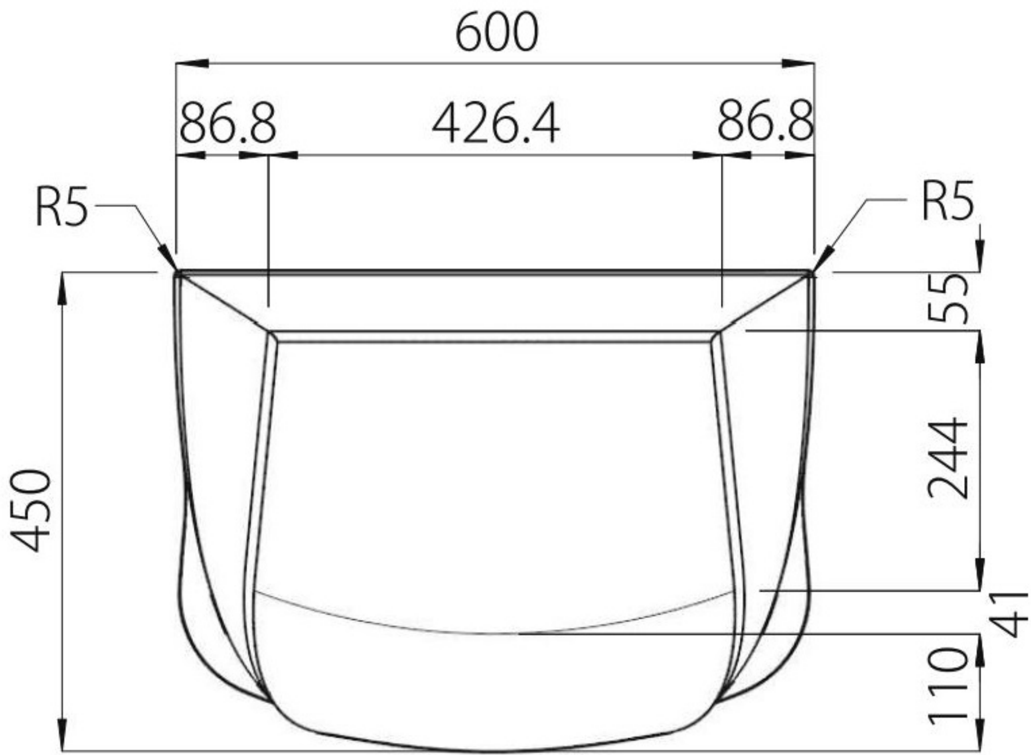
【平面図】
