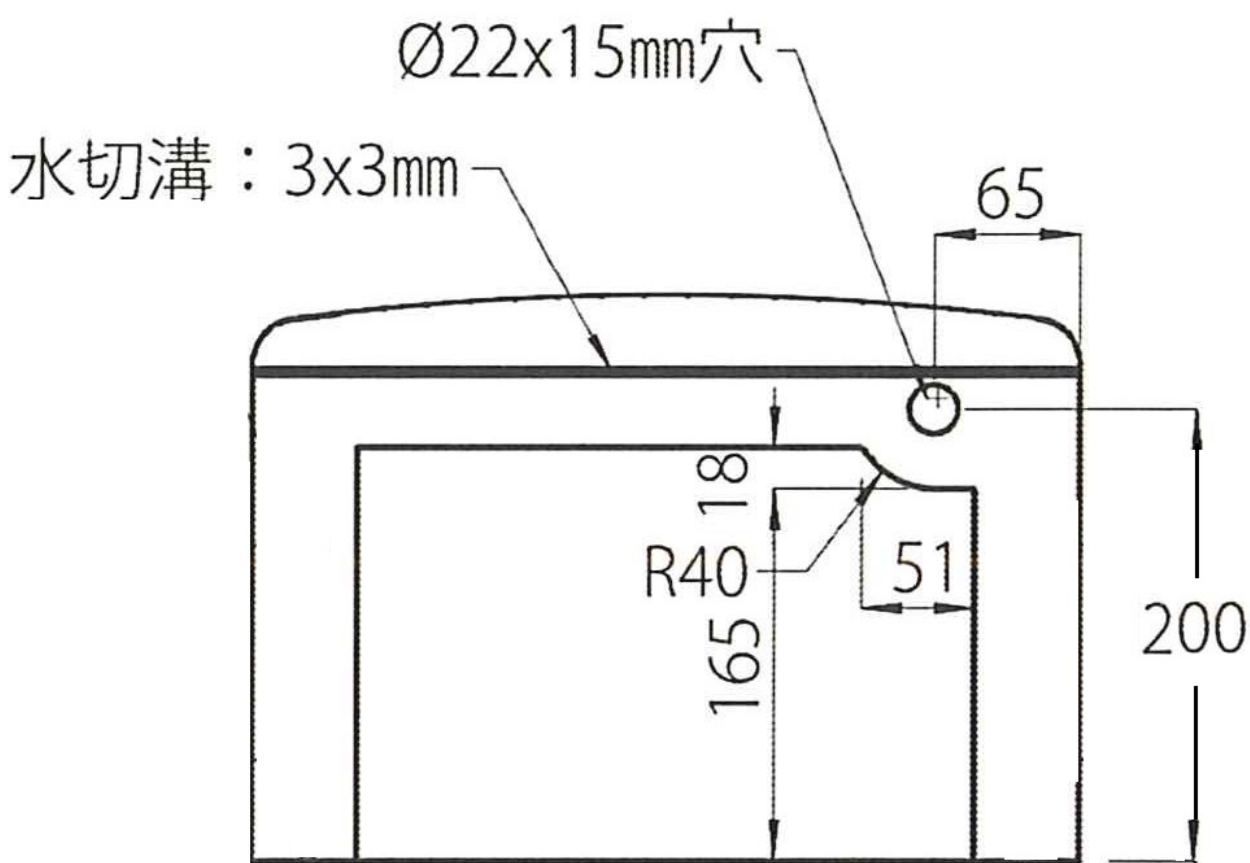
【底面図】
