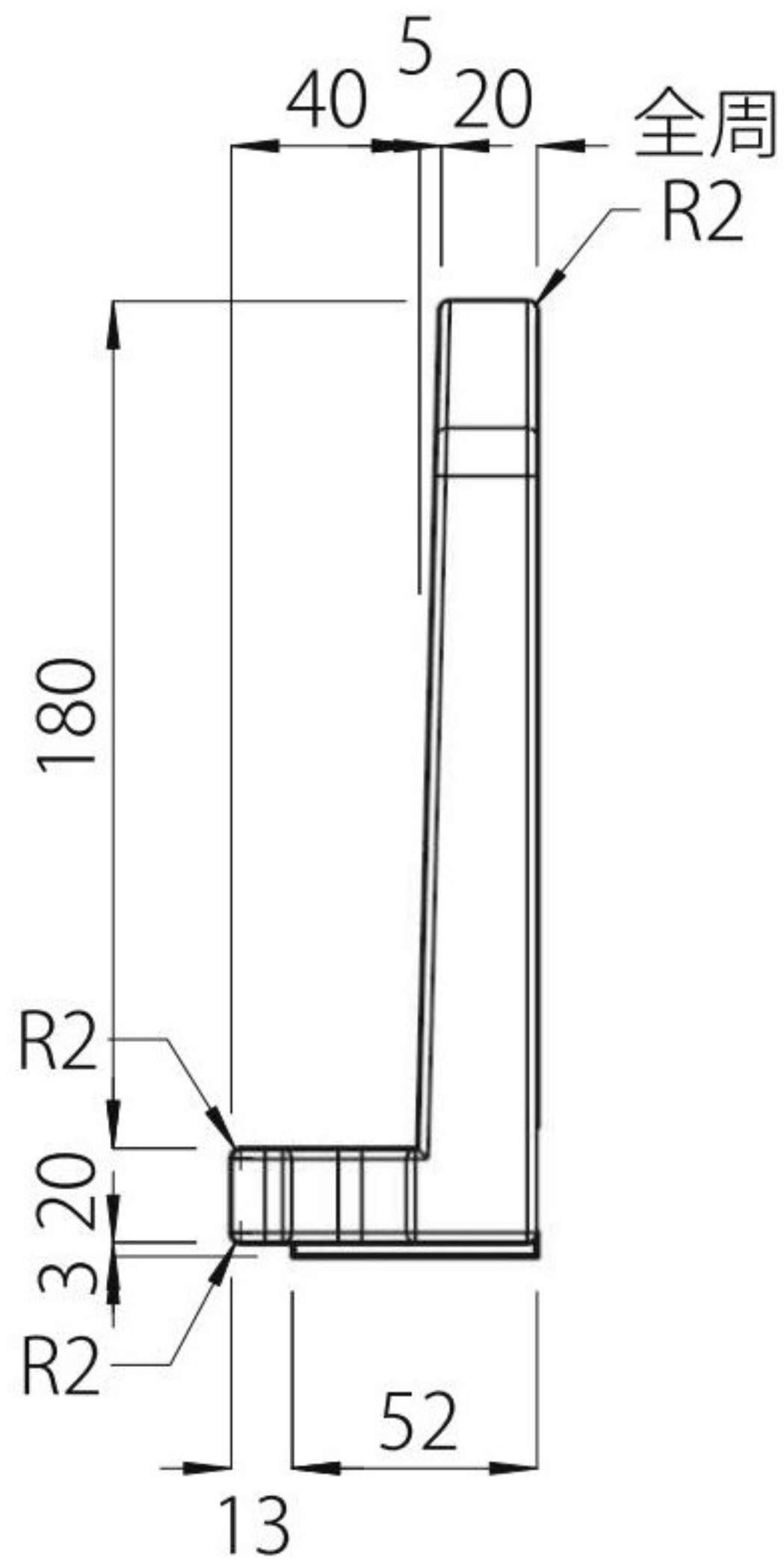
【右側面図】
