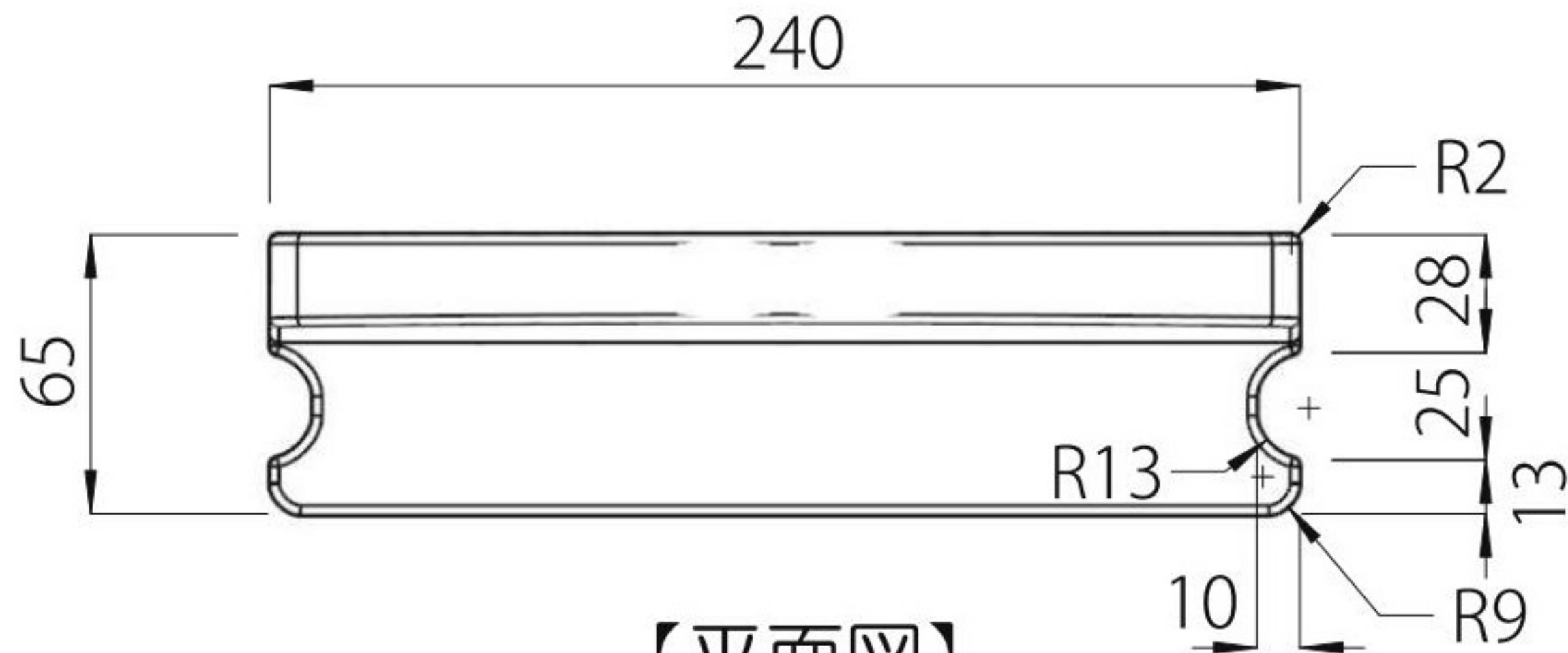
【平面図】
