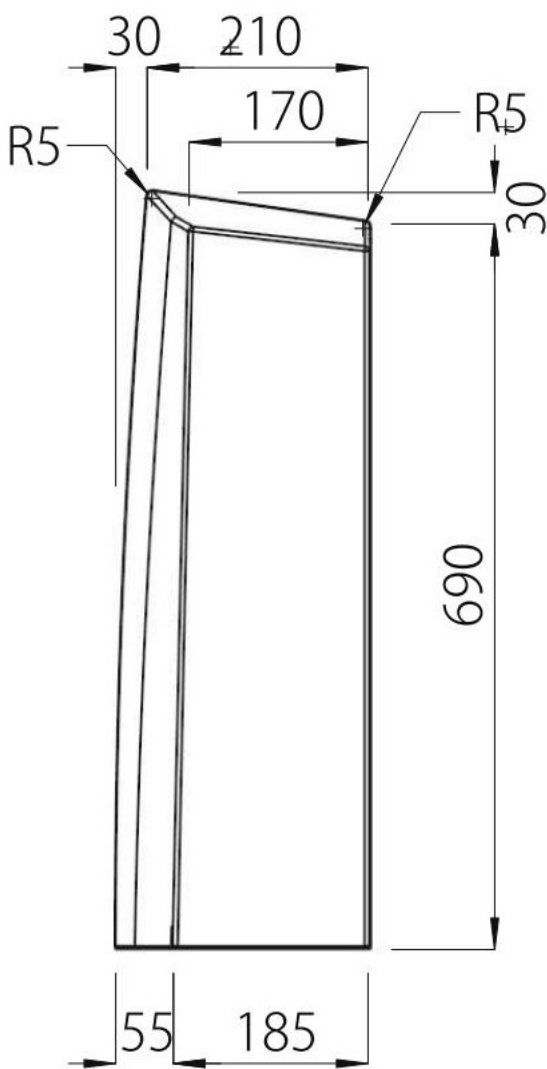
【右側面図】
