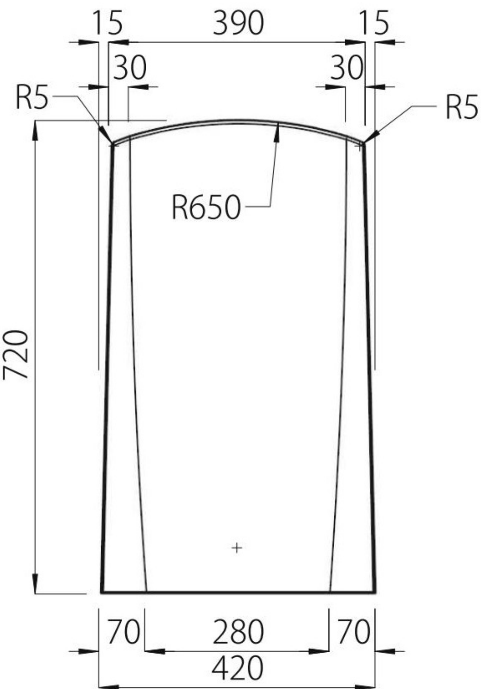
【正面図】
