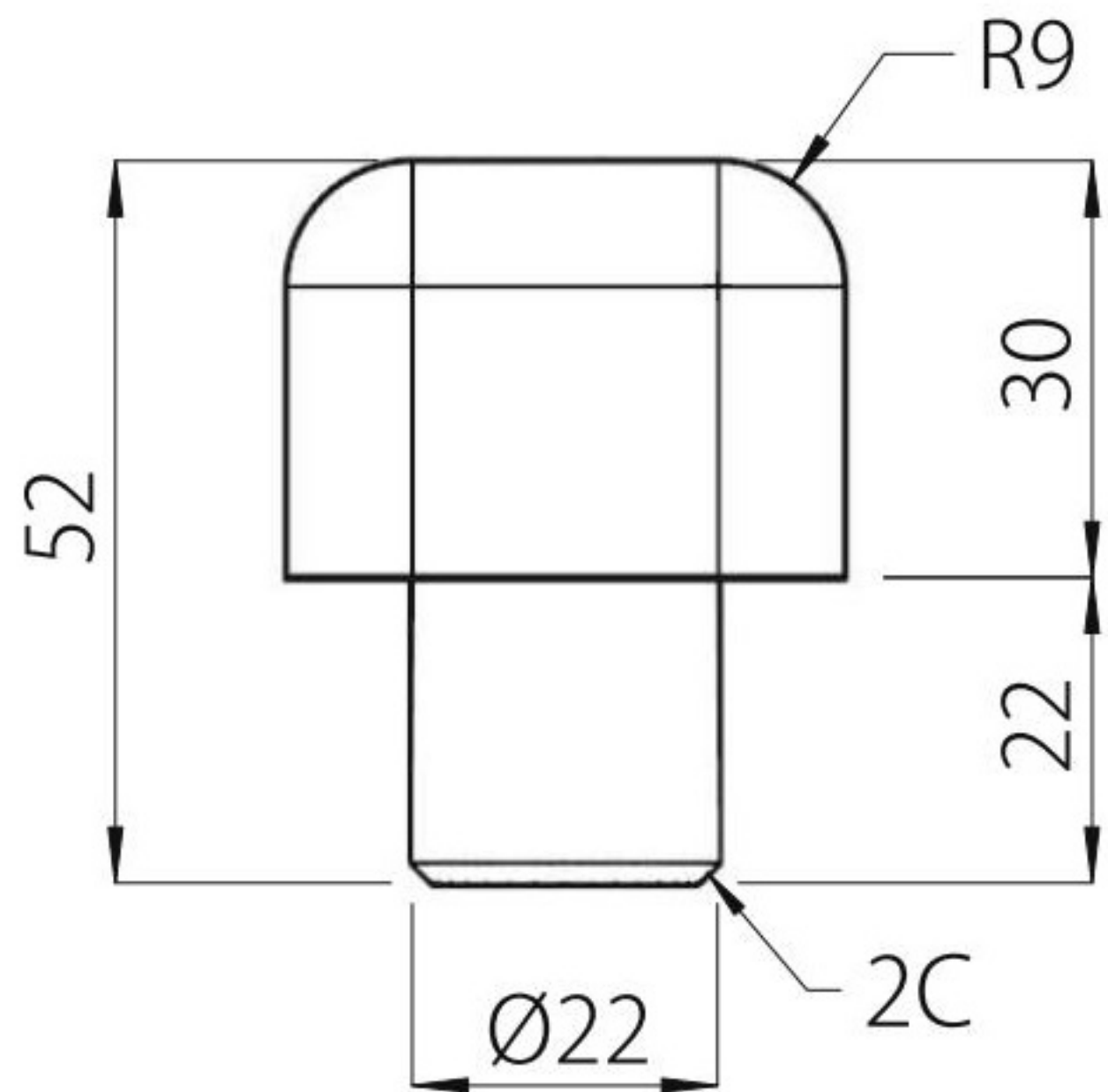
【正面図】
